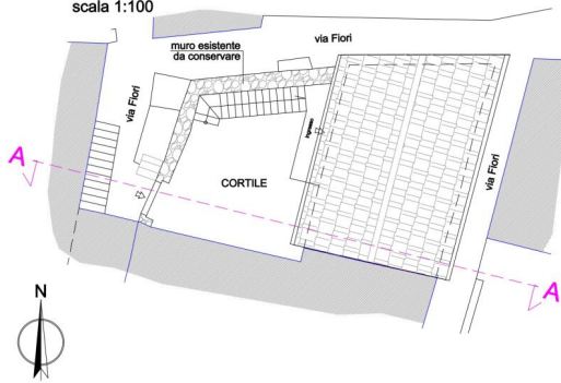
PLANIMETRIA PROGETTO scala 1:100
