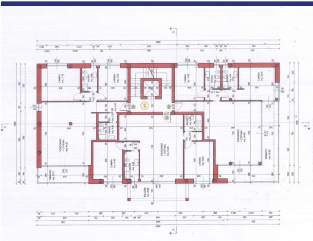
PIANTA PIANO PRIMO O. E.73
