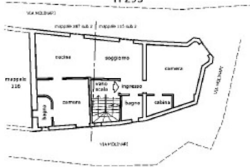
PIANTA PIANO TERRA H 275
