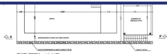
PIANTA PISCINA - scala 1:100
