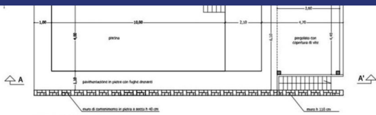
PIANTA PISCINA - scala 1:100
