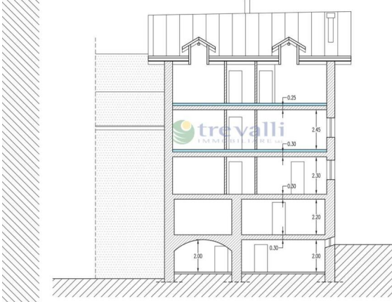
SEZIONE A/A
