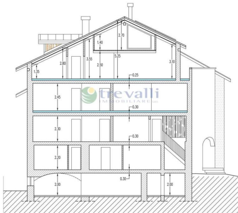
SEZIONE B/B
