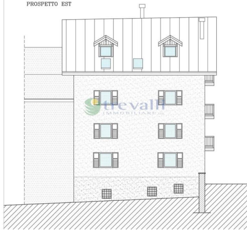
PROSPETTO EST
