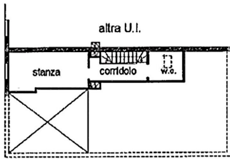
PIANO TERZO sottotetto h=2.20 med.
