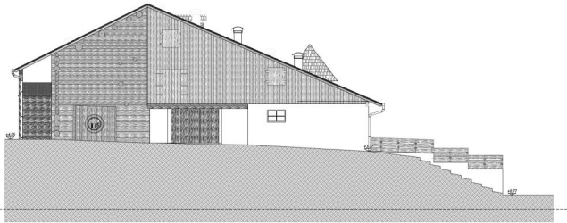
PROGETTO PROSPETTO_NORD
