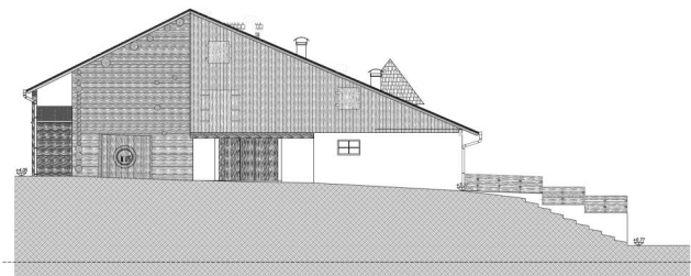
PROGETTO PROSPETTO_NORD
