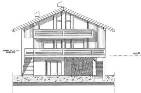
SEZIONE A-A PROGETTO sc. 1:100
